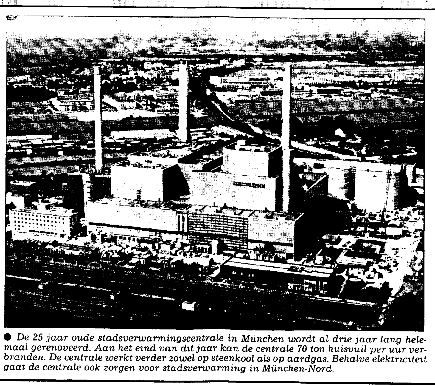
De 25 jaar oude stadsverwarmingcentrale in München wordt al drie jaar lang helemaal gerenoveerd. Aan het eind van dit jaar kan de centrale 70 ton huisvuil per uur verbranden. De centrale werkt verder zowel op steenkool als op aardgas.
